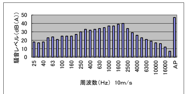
図-1 試験体No.1の風騒音レベル
