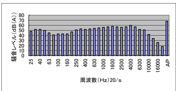
図-3 試験体No.3の風騒音レベル
