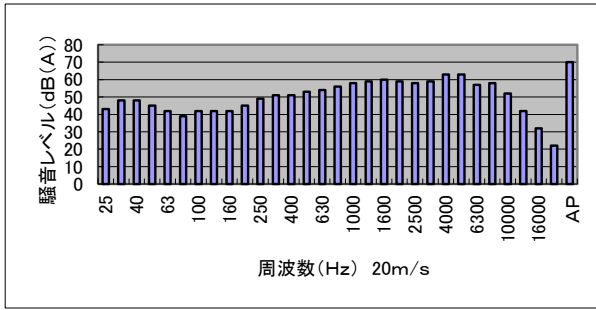
図-4 試験体No.4の風騒音レベル
