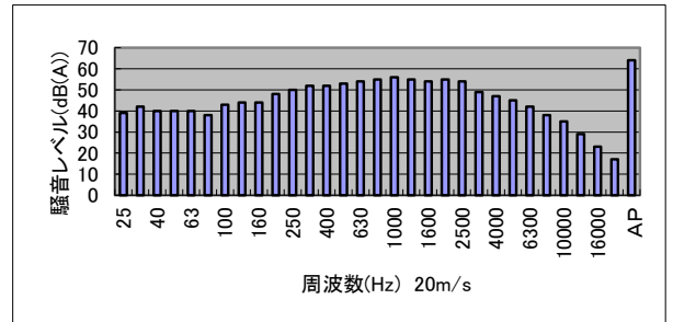
図-1 試験体No.1の風騒音レベル
