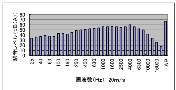
図-3 試験体No.3の風騒音レベル
