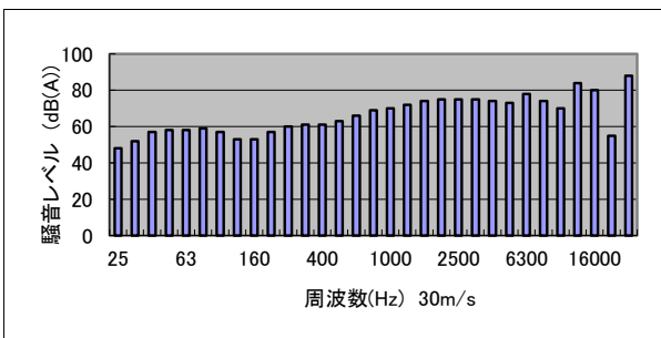
図-5 試験体No.5の風騒音レベル
