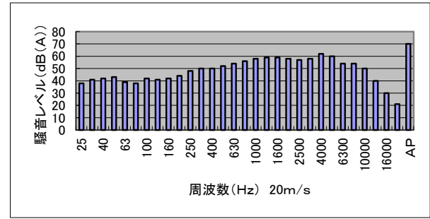
図-4 試験体No.4の風騒音レベル
